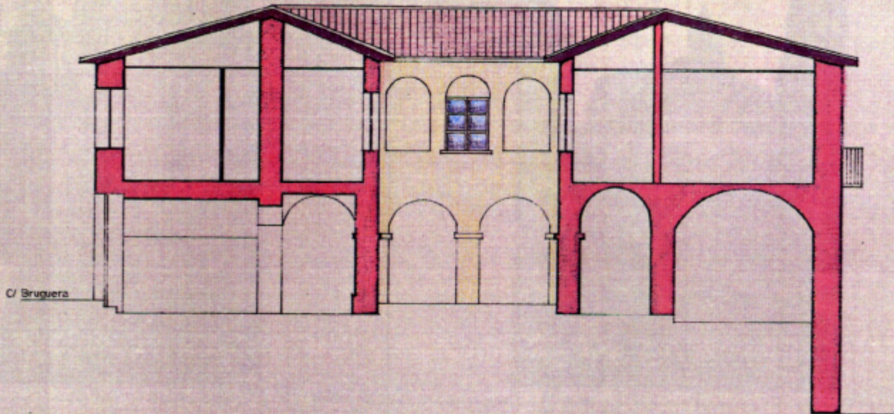
1. SECCION 1-1
