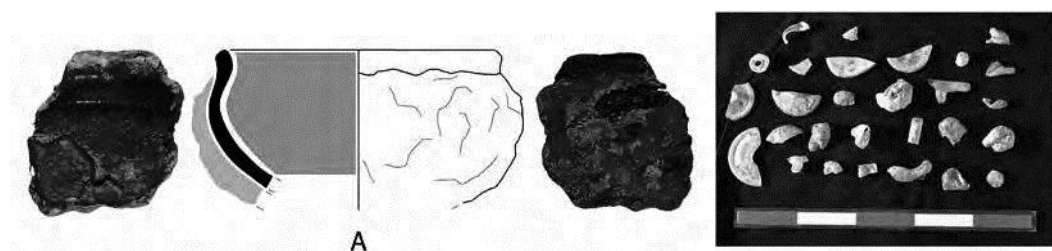
Figura 169. Dibuix i fotografies de la cassola de ceràmica de cuina utilitzada com a gresol de vidre. Fotografia dels fragments de copes de Foy 23a i dels rebuigs de vidre (extret de RODRÍGUEZ 2020).
