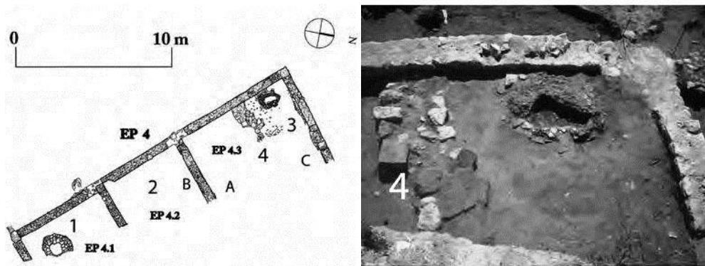
Figura 168. Planta de l'edifici productiu EP2 del suburbi portuari de Tarragona i fotografia de detall de l'àmbit 3 amb el forn de fusió del taller secundari de vidre (extret de RODRÍGUEZ 2020).
