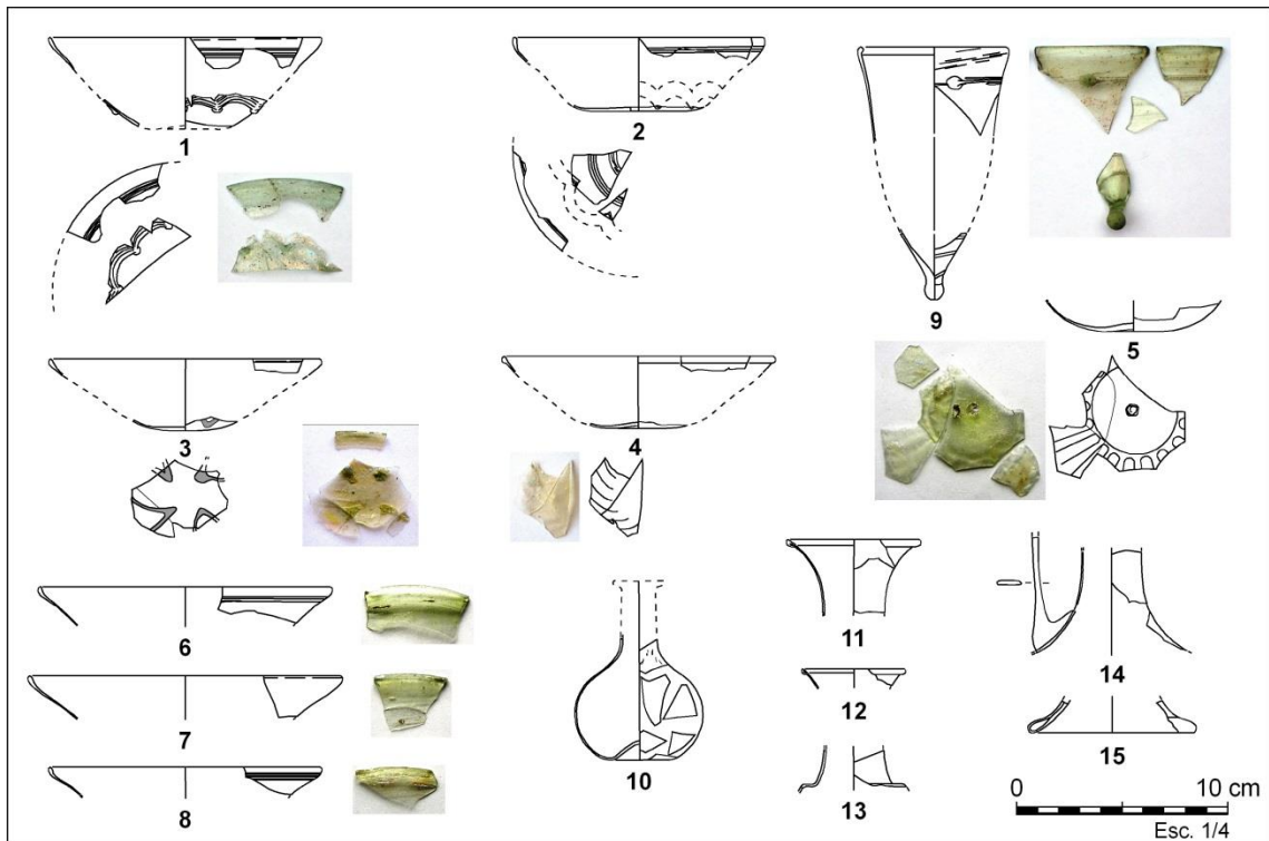
Figura 201. Recipients en ús a la Tarraconense Oriental (Catalunya i Andorra ) entre el 475/490 i el 530 AD, de producció verd aigua: 1-3, escudelles Foy 21a decorades amb fils de vidre blanc. 4-5, escudelles Foy 21a marcada en motlle amb costelles en relleu. 6-8, escudelles Foy 21a decorades amb fils de vidre blanc anellant la vora. 9, got cònic Foy 21c. 10, ampolla globular Foy 26. 11-13 ampolles cilíndriques Foy 25. 14-15, gerra amb nansa i peu tubular.
