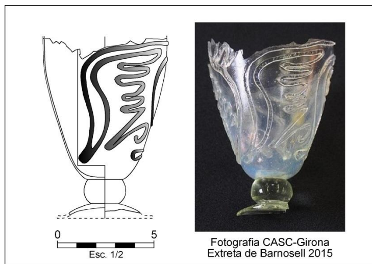
Figura 80. Derelict de d'Aiguablava VI (Begur), base de gerra Isings 93.
