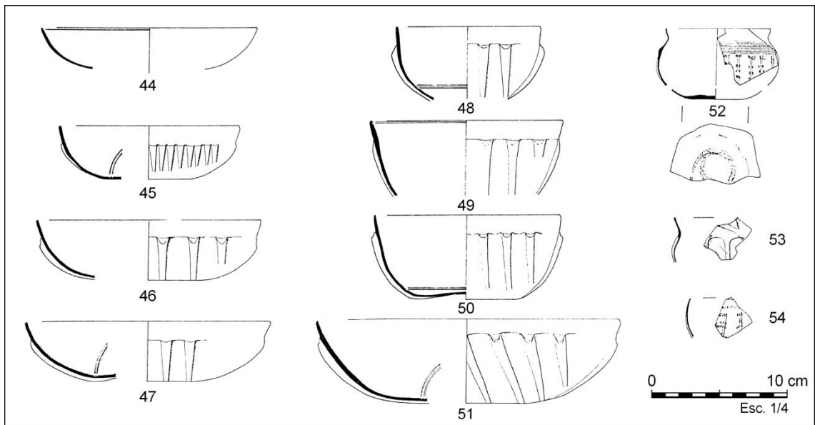
Figura 40. Passatge de Cobos (Tarragona): Vasos fosos en motlle: 44, ls. 1. 45-51, ls. 3. 52-54, ls. 17. Reelaborat de Price 1981.
