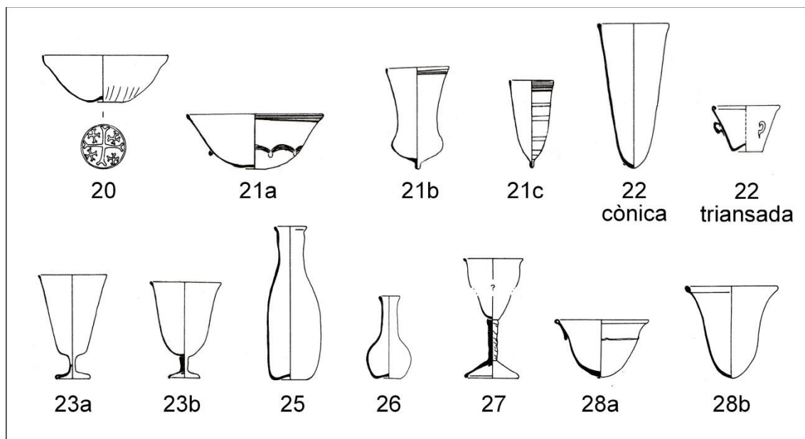
Figura 7. Tipologia de les formes de vasos de vidre definides per Danielle Foy i més comunes a l'època visigoda (s. VI-VIII) en el territori de la Tarraconense Oriental.
