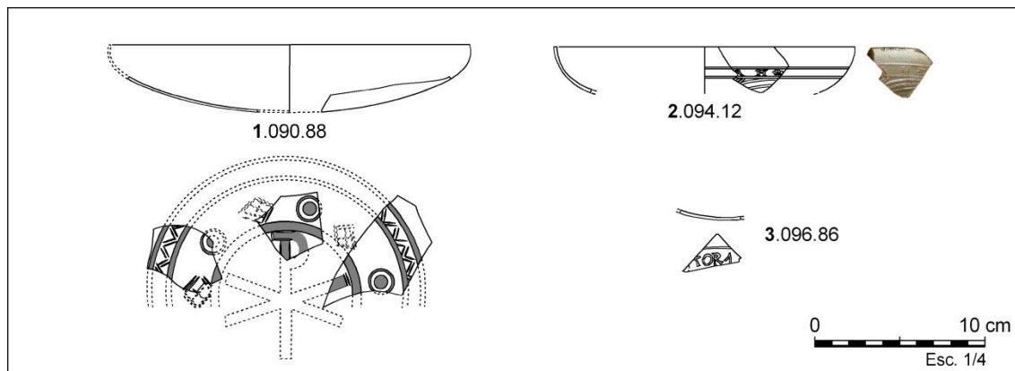
Figura 159. Escudelles Isings 116b gravades amb motius epigràfics: 1, Els Antigons (Reus). 2, C/ Vila-roma (Tarragona). 3, Necròpolis Paleocristiana -Fons Antic- (Tarragona).
