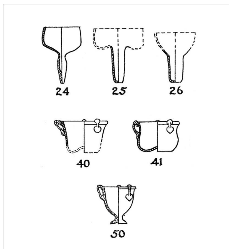
Figura 8. Tipologia de les llànties de vidre definides per Grace. M. Crowfoot i Donald B. Harden a Egipte i el mediterrani oriental, més comunes i del període visigòtic (s. VI-VIII) a la Tarraconense Oriental.
