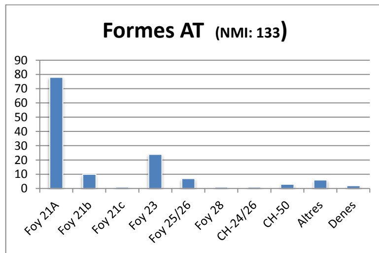
Figura 15. Vidre de C/ Sant Honorat 3 (Barcelona). NMI documentats per forma al període visigòtic.
