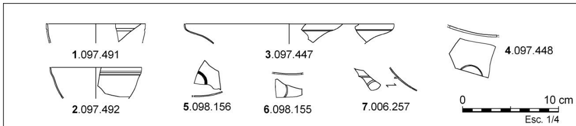
Figura 158. Copetes Is. 96b gravades amb motius lineals simples: 1 , Necròpolis Paleocristiana -Caixa 1987- (Tarragona). Escudelles Isings 116 gravades amb motius lineals simples: 3 i 4 , Necròpolis Paleocristiana -Caixa 1987- (Tarragona). 5 i 6 , Parcel·la 22b del PERI 2 (Tarragona). 7 , Pla de Palol (Platja d'Aro)
