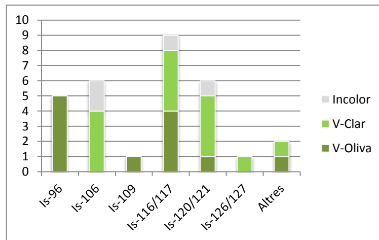
Figura 10. NMI dels tipus formals del baix imperi
