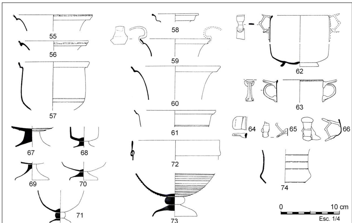
Figura 41. Passatge de Cobos (Tarragona): Vasos bufats: 55-61, Cantharos ls. 38. 62-66, skyphos ls. 39. 67-70 tiges massisses de carchesium o cantharos . 71. Tija globular de cantharos ls. 38. 72, modiolus ls. 37. 73, peu amb tija globular de cantharos amb fils aplicats. 74, carchesium ls. 36. Reelaborat de Price 1981.
