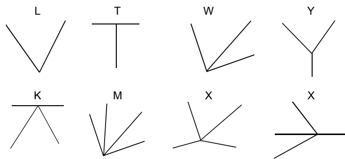
Figura 2-7. Tipos de uniones triédricas y tetraédricas
