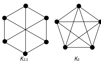
Figura 4-6. Grafos K_{3,3} y K_5 .
