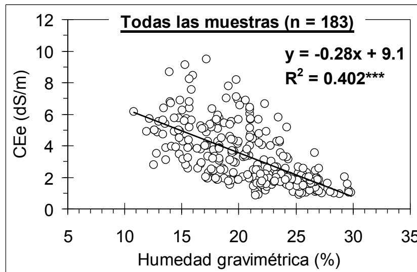
Figura IV.96. Regresión lineal entre la salinidad (CEe) y humedad gravimétrica (HG) del suelo para el total de muestras tomadas en los años 2010 a 2012 en el ensayo de nectarina en Caspe.
