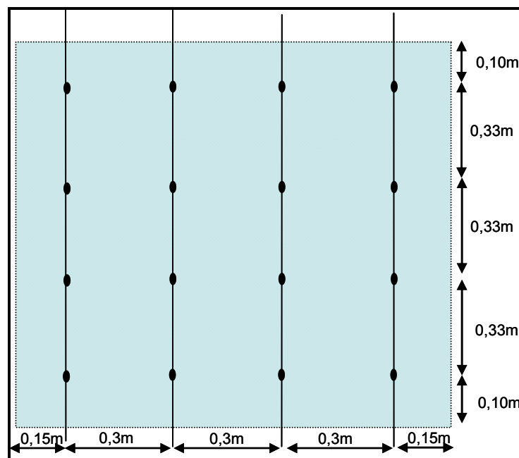
Figura III.6. Esquema de la situación de los 16 goteros en cada una de las miniparcelas de 1.2 m x 1.2 m del ensayo de evaporación en campo.
