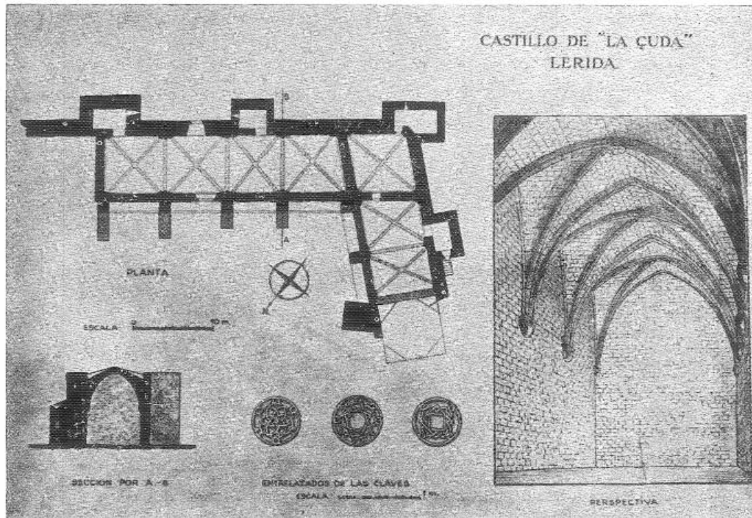
Fig. 44. Plànols i perspectiva interior amb les voltes i el elements sustentants de la coberta de la nau sud, Castell del Rei de Lleida.
