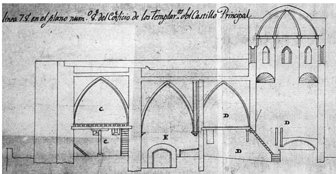
Fig. 42. Secció longitudinal de l'ala occidental del Castell del Rei de Lleida, 1796.
