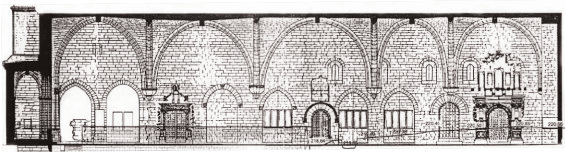
Fig. 36. Alçat de la façana sud de la Canonja.
