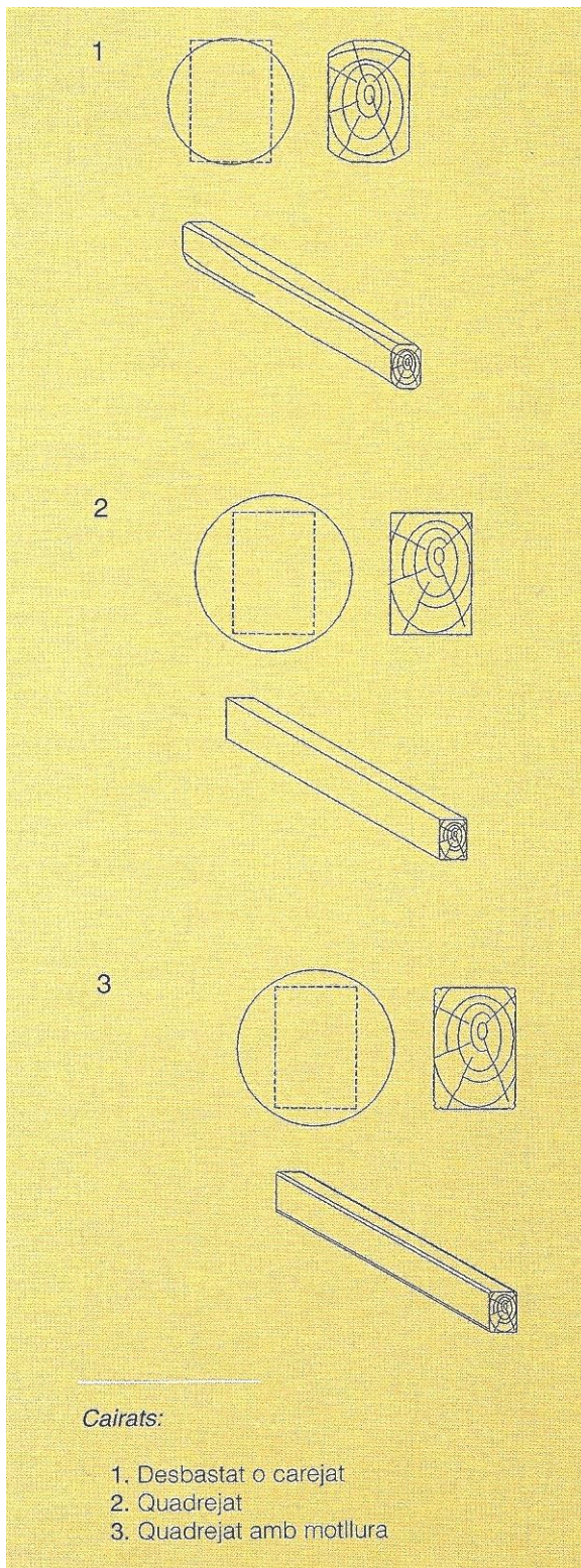
Imatge 25: Tipus de talla de les bigues i cairats: desbastat o carejat, quadrejat, quadrejat amb motllura. AA.DD. (2005: 99)
