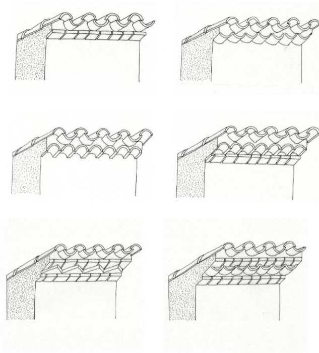
Imatge 41: Models de ràfecs de teulada. (Curós, J., 1993: 120-121)
