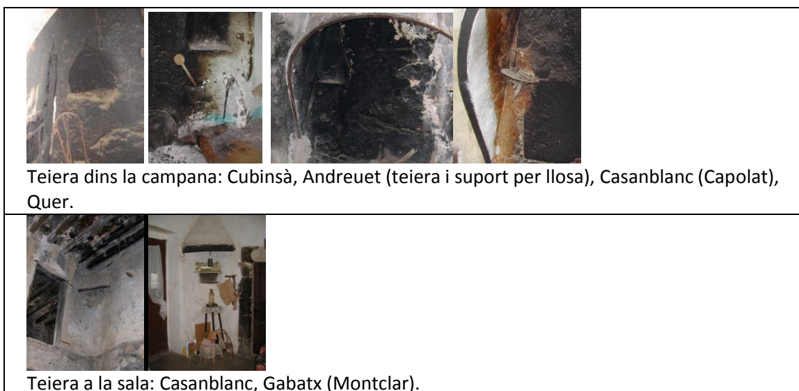
Imatge 98: Teieres dins la campana del foc.
