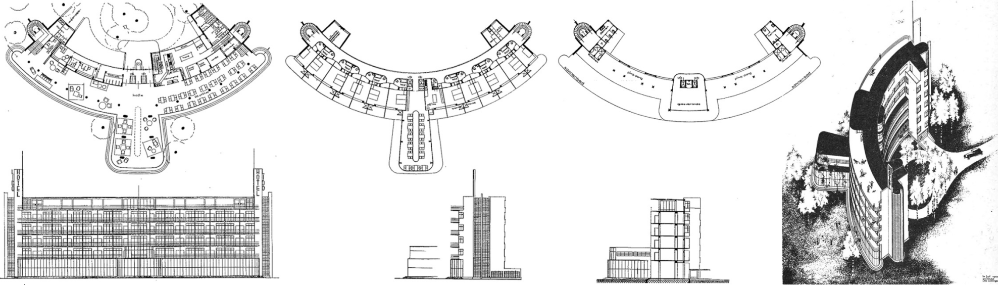
7 | 1931. Proyecto de Strand-Golf-Hotel. Ascona. Otto Zollinger "Progetto di albergo per il lido di Ascona". Alberghi di tutto il mondo: alberghi vecchi e nuovi, insegne di albergo, Domus (1940); pg. 58-59
