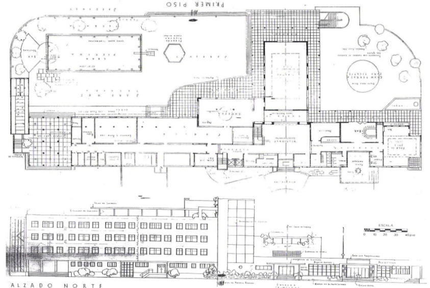
22 1945. Jaragua Hotel. Ciudad Trujillo. Guillermo González Sánchez "Hotel Nacional (Jaragua)" [c: 20.04.15] [d]: http://timerime.com/es/evento/1210217/Hotel+Nacional+Jaragua/ || "Hotel Jaragua" [c: 20.04.15] [d]: http://imagenesdenuestrahistoria.com/2013/04/07/hotel-jaragua/
