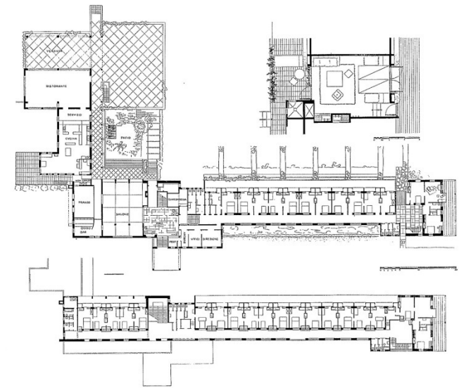
17 | 1938. Hotel Kalia. Mar Muerto. Zeev Rechter "Albergo Callia sul Mare Morto" Alberghi di tutto il mondo: alberghi vecchi e nuovi, insegne di albergo, Domus (1940); pg. 66-67 || "The Kalia Hotel at the Dead Sea" [c: 19.02.15] [d]: http://www.rechter-arch.com
