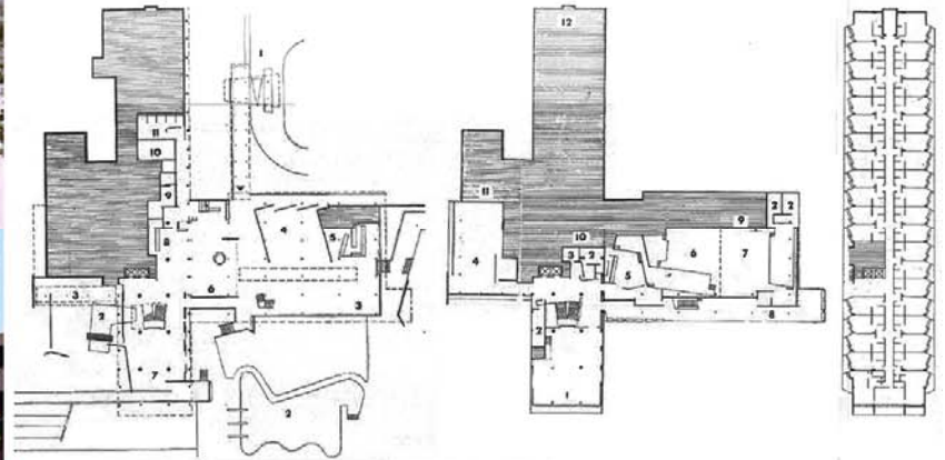
27 | 1949. Hotel Caribe Hilton. San Juan de Puerto Rico. Oswaldo Toro, Miguel Ferrer y Luis Torregrosa. "The Caribe Hilton Hotel", L'Architecture d'Aujourd'hui n.º 40 (abril, 1952), pg. 2-5 || "CARIBE-HILTON" [c: 20.04.15] [d]: http://www.ebay.es/itm/VINTAGE-POSTCARD-CARIBE-HILTON-HOTEL-SAN-JUAN-PUERTO-RICO-1950s-
