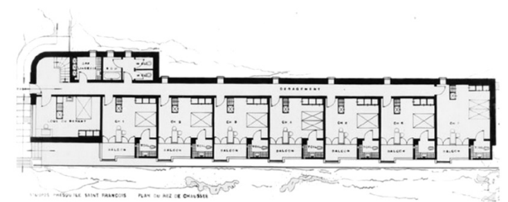
PROJET D'HOTEL SAINT FRANCOIS PLAN DU RIZ DE CHASSE
