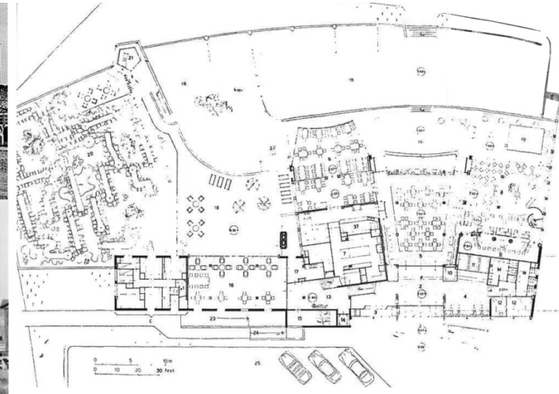
36 | 1952. Hotel Bouwes. Zandvoort. Jan Wils "Seaside hotel at Zandvoort" L'Architecture d'Aujourd'hui , nº 61 (1955, setiembre), pg. 21 || "Het oude Hotel Bouwes" [c: 26.04.15] [d]: http://www.freewebs.com/oud-zandvoort/toudehotelbouwes.htm
