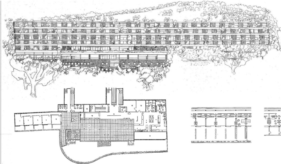
13 | 1937. Proyecto de Hotel Nord-Est. Isla de Santa Margherita. Luigi Vietti . "Albergo Nor-est". Alberghi di tutto il mondo: alberghi vecchi e nuovi, insegne di albergo, Domus (1940) ; pg. 18-19
