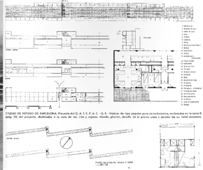
11 | 1932. Hoteles de tipo popular para la Ciudad de Reposo. Barcelona. GATEPAC . Documentos de Actividad Contemporánea. "La ciudad de reposo que necesita Barcelona". nº7 (julio-setiembre, 1932), pg. 24-31 y "Exposición de La Ciudad de Reposo de Barcelona" nº 13 (enero-marzo, 1934) pg. 23-28
