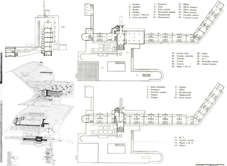
9 | 1932. Hotel Latitude 43. Saint Tropez. Georges-Henri Pingusson . "Albergo Latitude 43 a S. Tropez. Francia". Alberghi di tutto il mondo . Domus. Milan, (1940) pg. 45-51 || Cité de l'architecture et du patrimoine [ol] [c: 09.02.20] [d]: http://www.citechallot.fr/ressources/expositions_virtuelles/vegetal/03-
