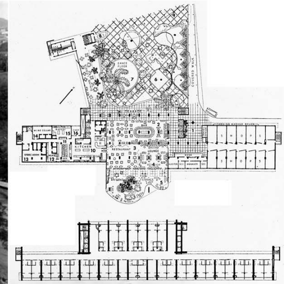
31 | 1950. Hotel Ofir. Ofir. Alfredo Ângelo de Magalhães LOBO, S. L. M.: "Arquitectura e Turismo: Planos e Projectos. As Cenografias do Lazer na Costa Portuguesa. Da 1.ª República à Democracia" [c: 25.04.15] [d]: https://estudogeral.sib.uc.pt/handle/10316/23799
