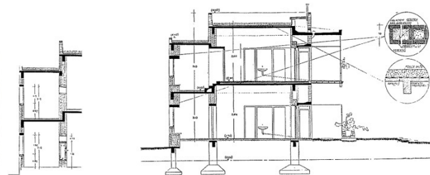
17 | 1938. Hotel Kalia. Mar Muerto. Zeev Rechter "Albergo Callia sul Mare Morto" Alberghi di tutto il mondo: alberghi vecchi e nuovi, insegne di albergo, Domus (1940); pg. 66-67 || "The Kalia Hotel at the Dead Sea" [c: 19.02.15] [d]: http://www.rechter-arch.com
