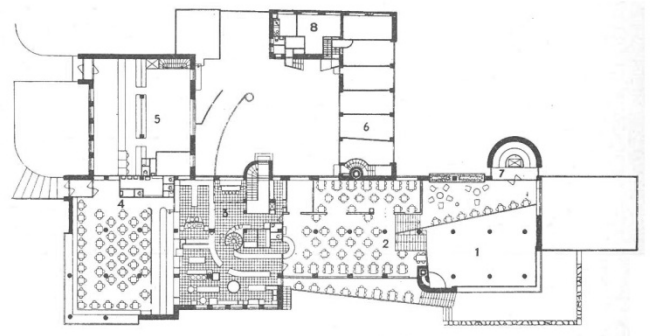
16 | 1937. Hotel Pohjanhovi. Rovaniemi. Pauli Ernesti Blomstedt "Un albergo al Circolo Polare Artico" c. 09.02.19 [d]: http://www.casadellarchitettura.eu/fascicolo/data/2011-03-25_438_1918.pdf || [c: 19.02.15] [d]: http://archinfo.fi/2014/05/vaitos-lapin-matkailurakentamisesta
