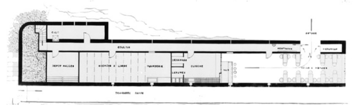
PROJET D'HOTEL SAINT FRANCOIS PLAN DU RIZ DE CHASSE
