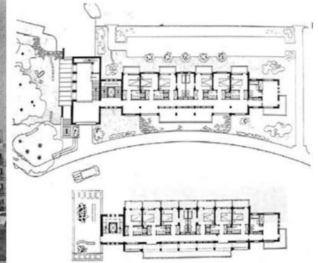
31 | 1950. Hotel Ofir. Ofir. Alfredo Ângelo de Magalhães LOBO, S. L. M.: "Arquitectura e Turismo: Planos e Projectos. As Cenografias do Lazer na Costa Portuguesa. Da 1.ª República à Democracia" [c: 25.04.15] [d]: https://estudogeral.sib.uc.pt/handle/10316/23799
