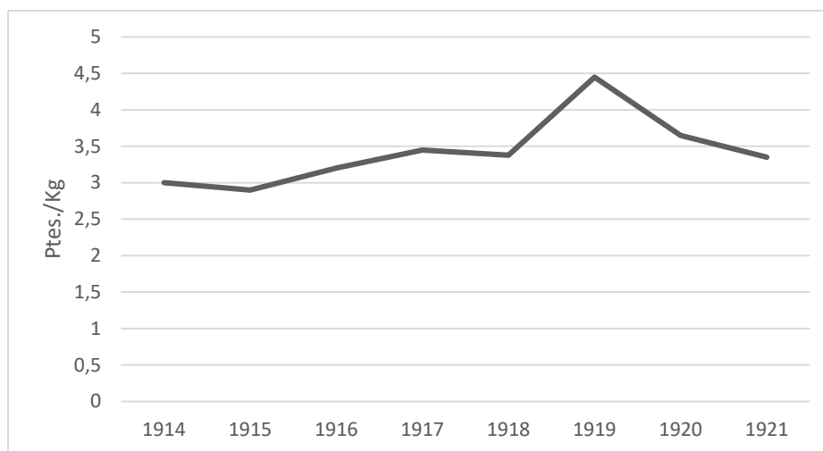
Figura 7. Evolució dels preus de cacau al port de Barcelona, 1914-1921 (Ptes./Kg)
