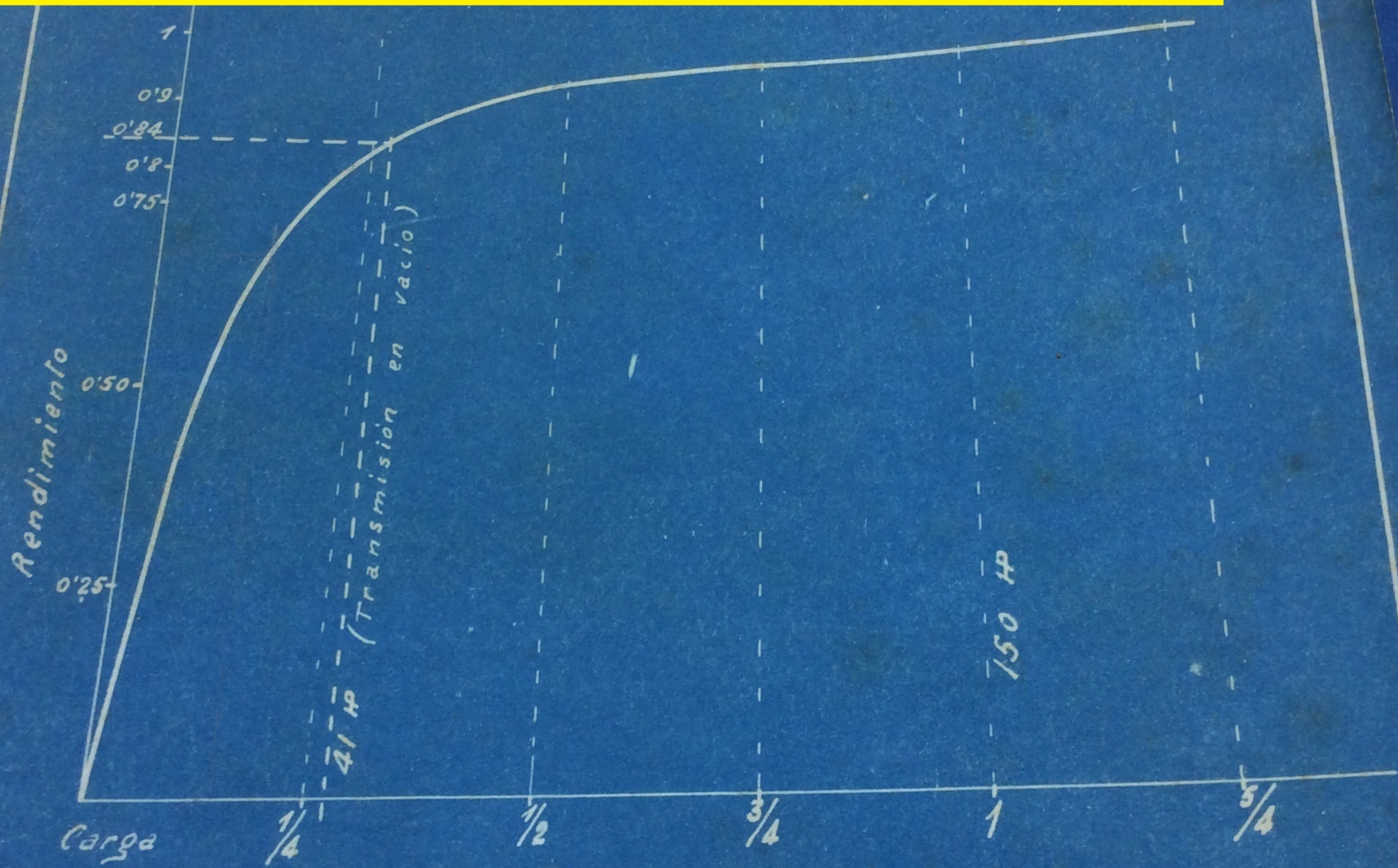
Característica del rendimiento de un motor trifásico de 150 HP
