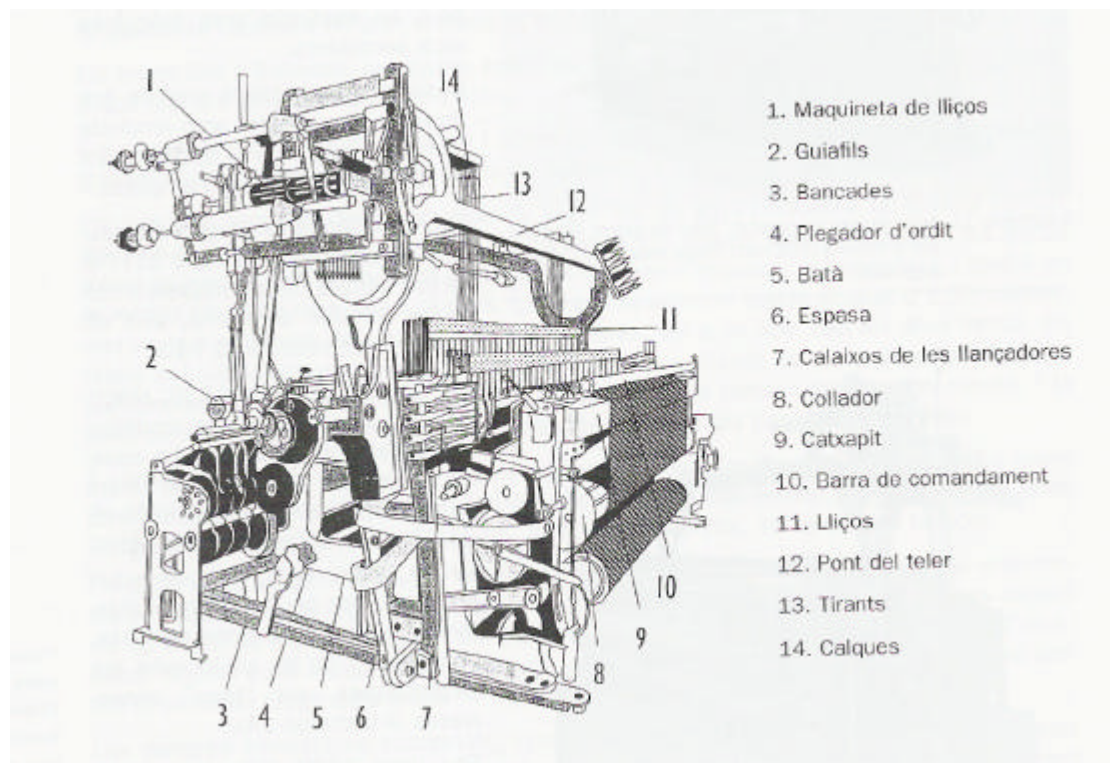
Imatge 18: Esquema d'un teler mecànic
