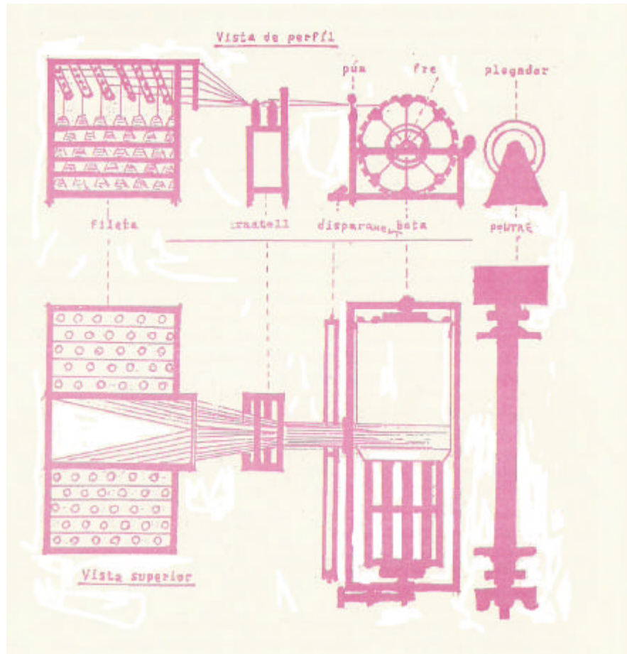
Imatge 15: Ordidor de bóta
