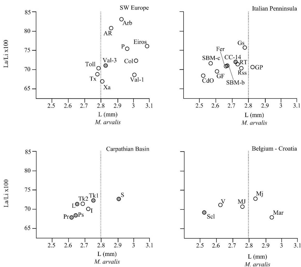
Figure 4.2.2. Relation between L and the La/Li index in Microtus arvalis of Late Pleistocene. In grey: MIS 5 samples. SW Europe : Val-3: Valdavara-3; Col: Colomera; Xa: Xaragalls; Tx: Teixonerres; P: Portalon; AR: Romaní (level O); Val-1: Valdavara-1; Arb: Arbreda. Italian Peninsula (I): CC-14: Ciota Ciara, unit 14; SBM-b: Grotta Maggiore di San Bernardino, units V-IV; SBM-c: Grotta Maggiore di San Bernardino, units III-II; CdO: Caverna degli Orsi; GF: Fumane; RSS: Roccia San Sebastiano; Fer: Ferrovia; GS: Grotta del Sambuco; RT: Riparo Tagliente; GP: Grotta Paglicci. Carpathian Basin (CB): S: Süttő 6; Ps: Poroslyuk cave; Pr: Porlyuk cave; L: Lambrecht cave; Tk1: Tokod, levels 4-6; Tk2: Tokod, levels 1-3; I: Istállóskő. Belgium (B): Scl: Scladina; MJ: Marie-Jeanne. Croatia (HR): V: Vindija; Ma: Marlera I; Mj: Mujina.
