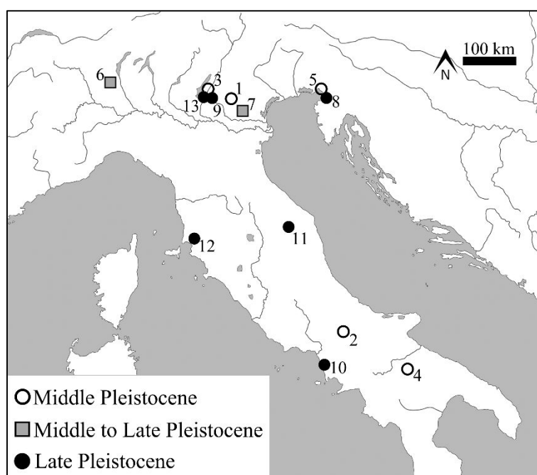
Figure 1. Geographical location of the sites. 1 = Spessa 10; 2 = Isernia; 3 = Bus de la Fadanana; 4 = Notarchirico; 5 = Visogliano; 6 = Ciota Ciara; 7 = Grotta Maggiore di San Bernardino; 8 = Caverna degli Orsi; 9 = Grotta Fumane; 10 = Roccia San Sebastiano; 11 = Grotta della Ferrovia; 12 = Grotta del Sambuco; 13 = Riparo Tagliente. White: Middle Pleistocene; grey: Middle to Late Pleistocene; black: Late Pleistocene.
