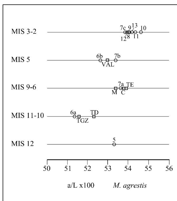
Figure 10. Variations in a/L index of M. agrestis . Circle = sample from the Italian Peninsula. MIS 12: 5 = Visogliano. MIS 11-10: 6a = Ciota Ciara; MIS 9-6: 7a = Grotta Maggiore di San Bernardino. MIS 5: 6b = Ciota Ciara, 7b = Grotta Maggiore di San Bernardino; MIS 3-2: 7c = Grotta Maggiore di San Bernardino (MIS 3) 8 = Caverna degli Orsi; 9 = Grotta Fumane; 10 = Roccia San Sebastiano; 11 = Grotta della Ferrovia; 12 = Grotta del Sambuco; 13 = Riparo Tagliente. Square = samples from southwestern Europe. TD = Trinchera Dolina; TGZ = Galeria-Zarpazos; TE = Sima del Elefante; C = Carrière; M = Mollet; VAL = Valdavara-3.
