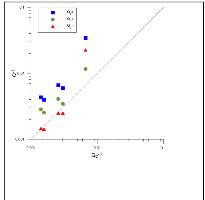
Figura A4.3.14.b Representación de los valores de Q_c^{-1} , Q_i^{-1} , Q_s^{-1} y Q_t^{-1} en función de Q_c^{-1} . De izquierda a derecha, las observaciones corresponden a las frecuencias 9Hz, 7Hz, 5Hz, 3Hz y 1.5Hz.
