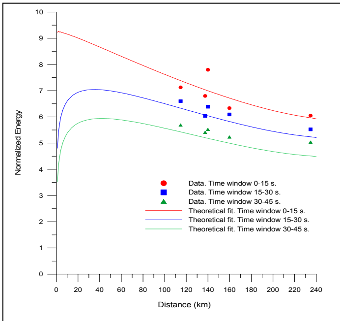
Figura A4.3.14.a Energía en función de la distancia hipocentral para la banda frecuencial 6-8 Hz. Ajuste entre energías teóricas (líneas continuas) y observadas.
