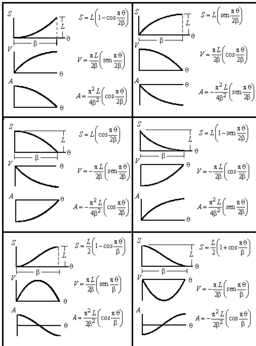
Figura A1-1 Leyes de desplazamiento con movimiento armónico. Tomado de Mabie y Reinholtz [2000]
