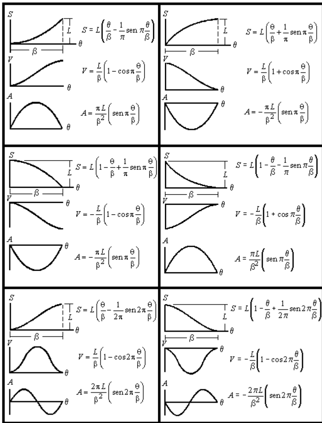
Figura A1-2 Leyes de desplazamiento con movimiento cicloidal. Tomado de Mabie y Reinholtz, [2000]
