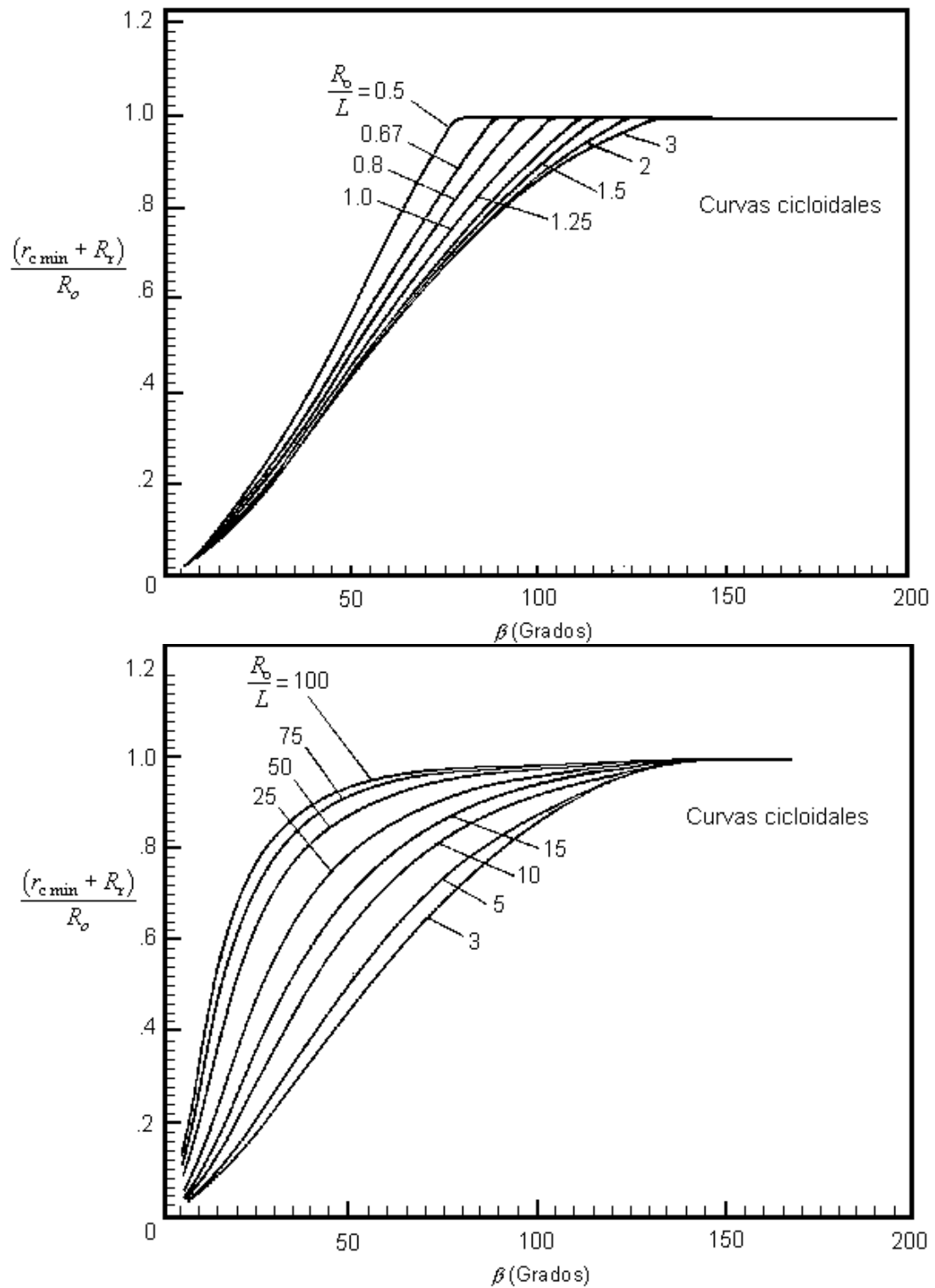
Figura A2-2 Radio de curvatura mínimo para levas con movimiento cicloidal de subida completa o de bajada completa. Tomado de Shigley y Uicker, [1988]
