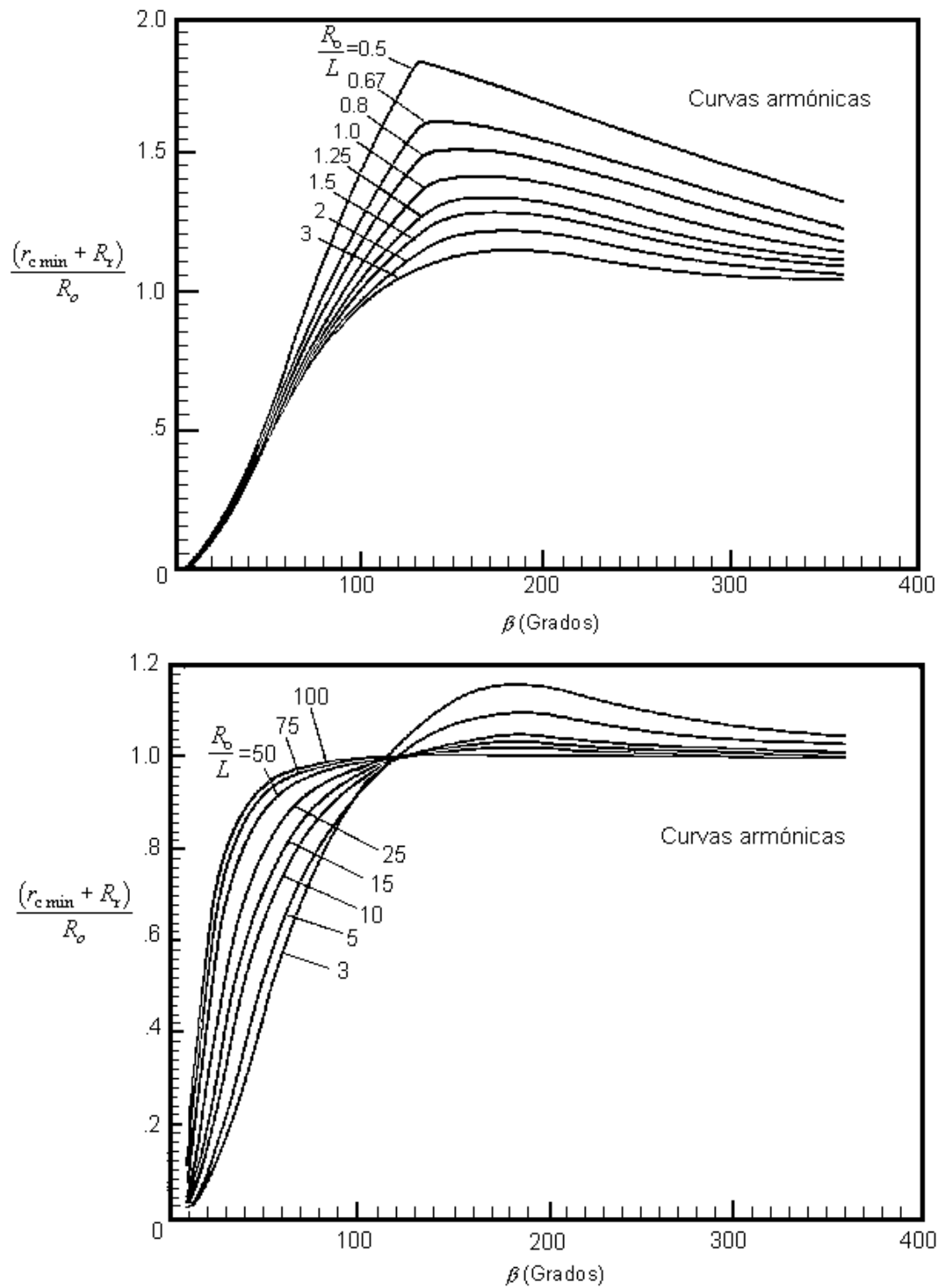
Figura A2-1 Radio de curvatura mínimo para levas con movimiento armónico de subida completa o de bajada completa. Tomado de Shigley y Uicker, [1988]
