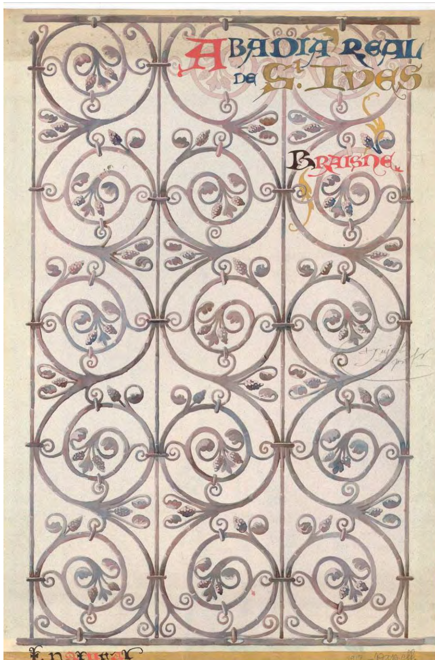
Proyecto: Rejas / Hierros artísticos / Abadies-Braise. Descripción: Abadía Real de St. Ives Braisne. Autor: Papell. Fecha: 1947 Escala: 1:1 Medidas: 94,5 x 63,3 cm. Biblioteca ETSAB: Nº inventario 5163 Cajón: 43 Técnica: Lápiz, tinta china y acuarela sobre papel. Notas: A la cara de la lamina: "t. natural". -- Firmado por el profesor Josep M.ª Jujol. – Reja.
