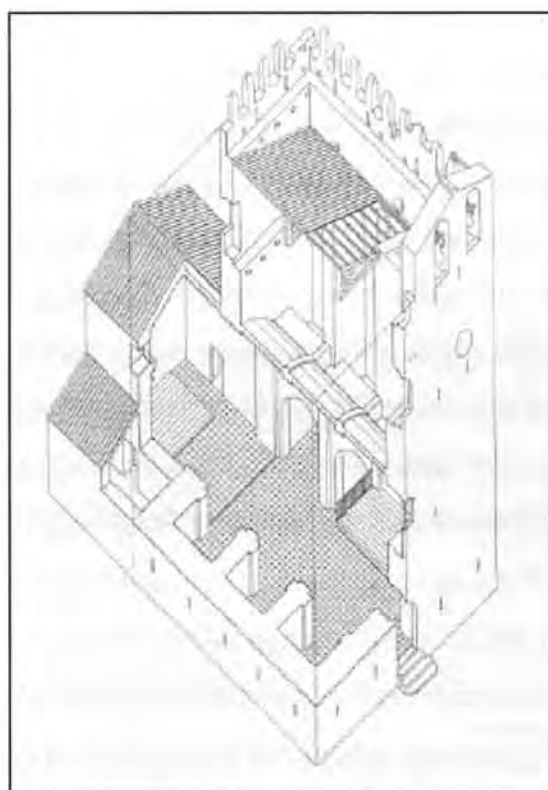
Axonometria de la torre de la Galera (Serveis de Patrimoni de la Generalitat)
