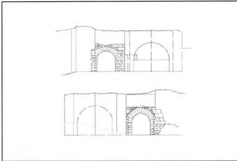
Alçat del portal de Tarragona (S. Viladrich)
