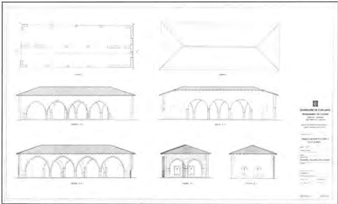
Planta i alçats de la llotja de Tortosa en la seua ubicació actual (Serveis territorials de Patrimoni de la Generalitat)
