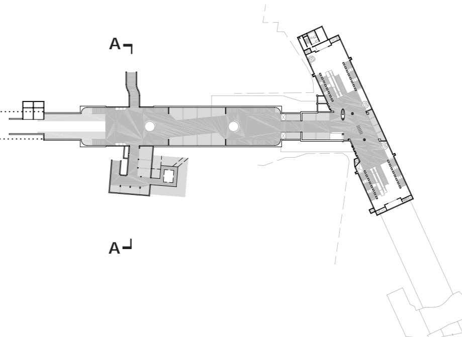
PLANTA MESANINA Y SALIDAS
