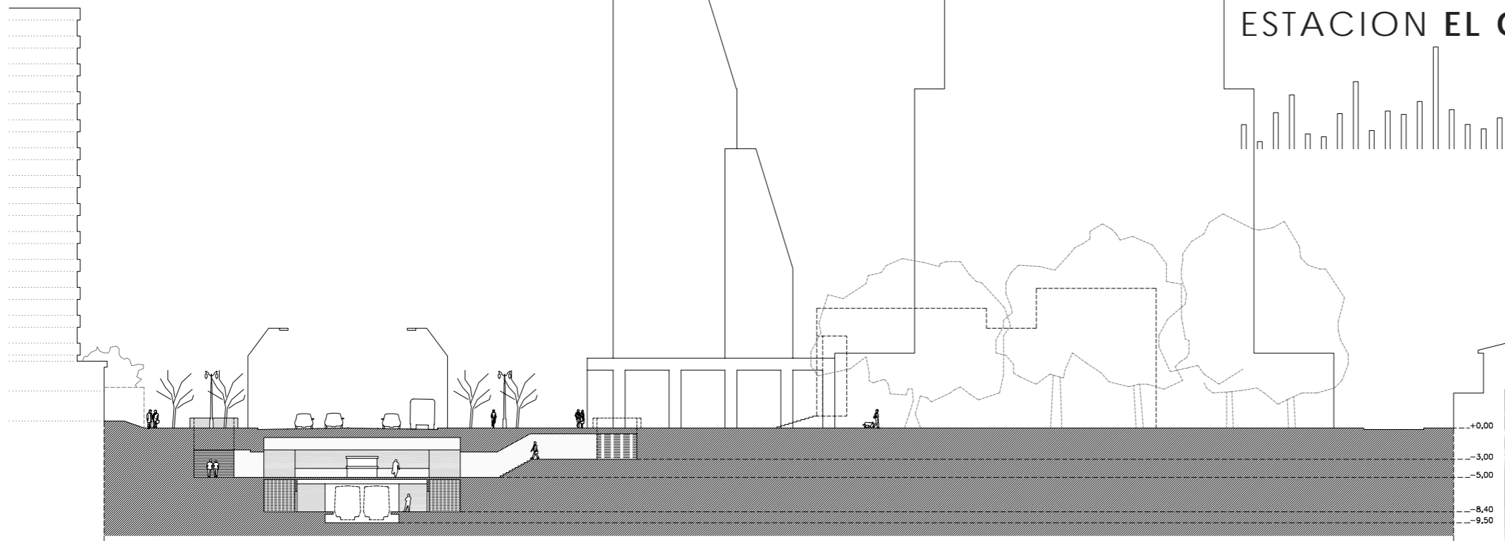
SECCION A-A
