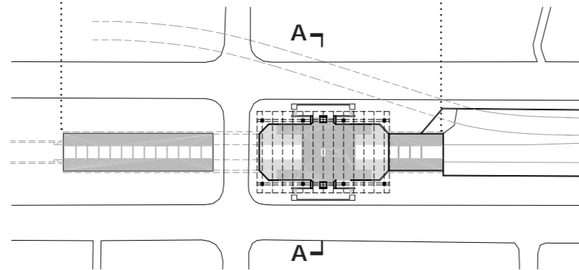
PLANTA MESANINA Y SALIDAS
