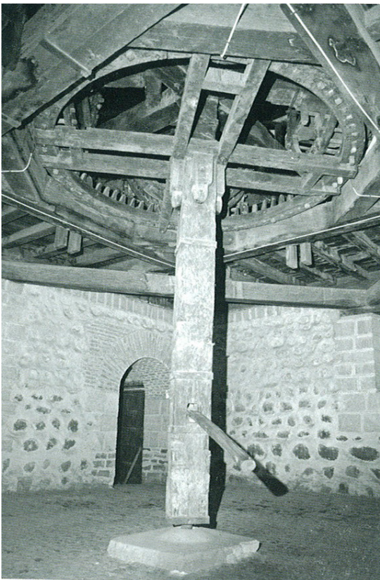
38. Part superior i inferior del molí de laminació mogut a sang de la Seca de Potosí, segle XVIII. Museo Casa de la Moneda, Potosí. Foto: projecte Euromint.
