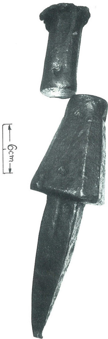
26. Joc de pila i trossell alemanys per encunyar moneda reproduïts a: COOPER. The Art and Craft , p. 28, segle XVI, Freiburg Museum.
