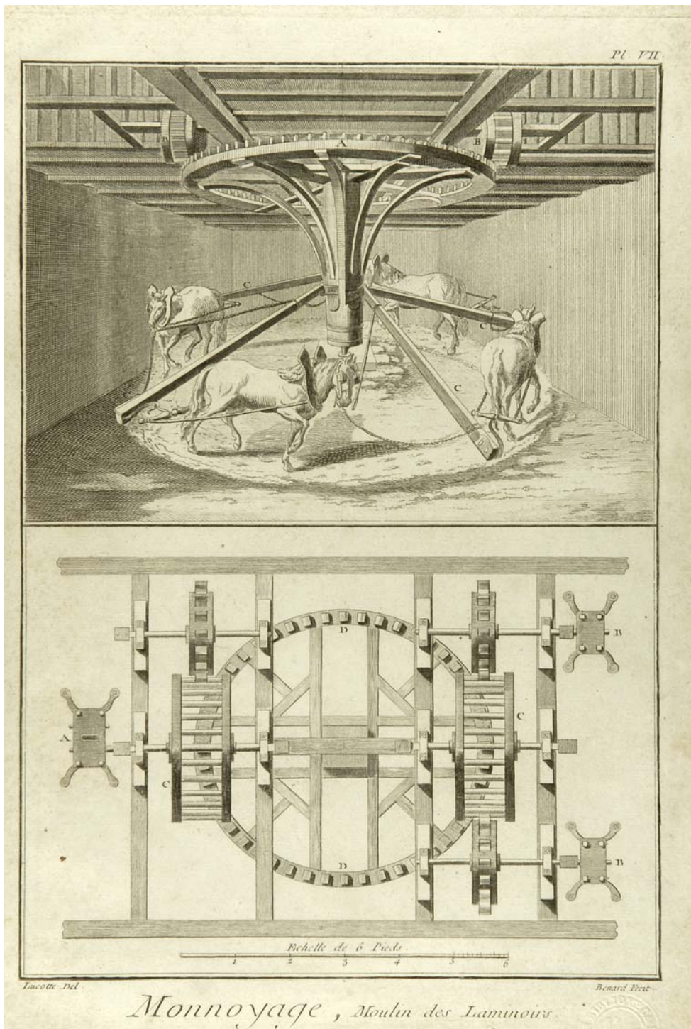
37. Molí mogut «a sang» destinat a laminar el metall que s'ha d'encunyar. Gravat que il·lustra l' Encyclopédie française , 1765. Biblioteca de Catalunya, Barcelona.
