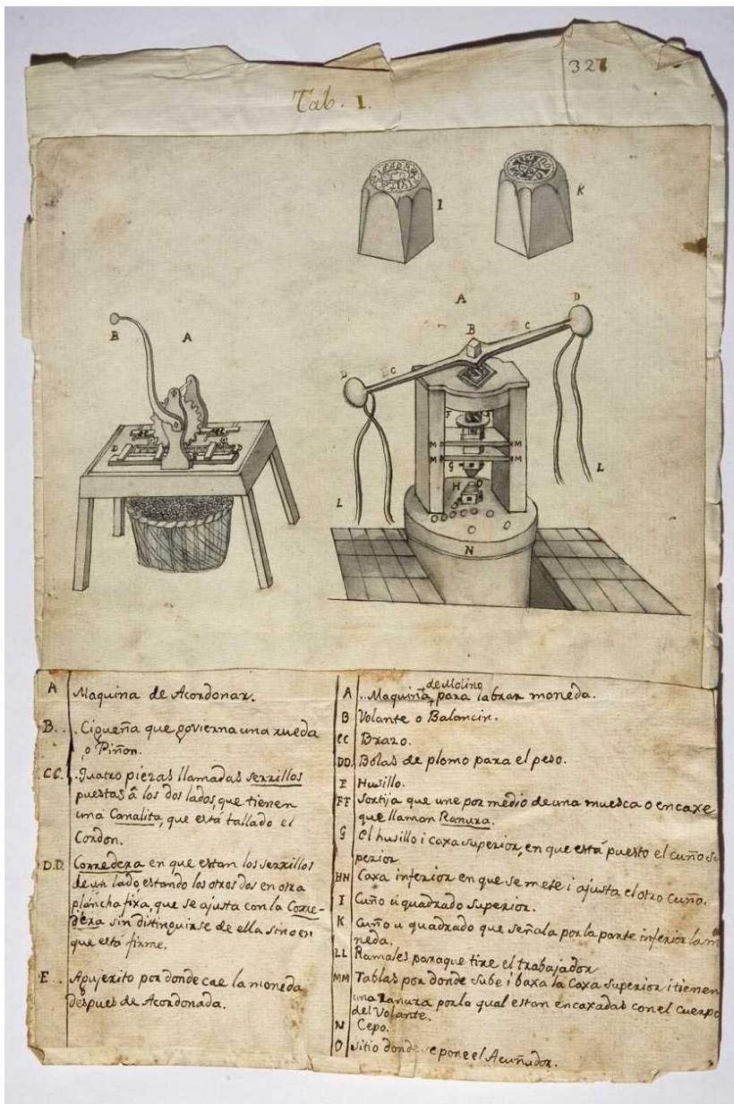
39. Dibuix anònim d'una màquina d'acordonar el cantell de la moneda i d'una premsa de balancí per a l'obra manuscrita de Josep Salat (1762-1832) Suplemento, o sea Continuación al Tratado de Medallas labradas en el Principado de Cataluña, con Documentos justificativos , primer quart del segle XIX. Reial Acadèmia de Bones Lletres Barcelona, Barcelona.
