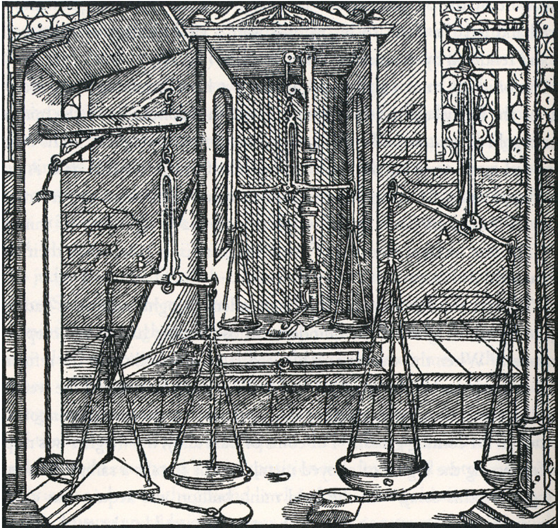
22. Diferents tipus de balances per pesar metall. Gravats que il·lustra l'obra de Georgius Agricola. De re metallica , 1556. Col·lecció particular, Barcelona.
